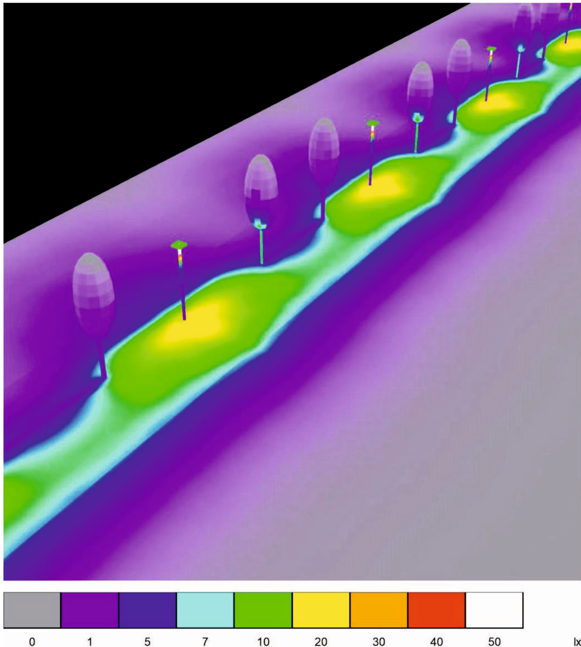
Набережная, торшерные светильники Фиктивные цвета — визуализация
